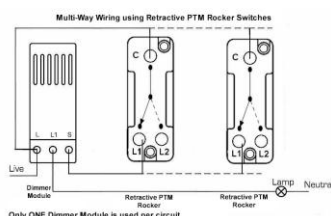
Wiring
